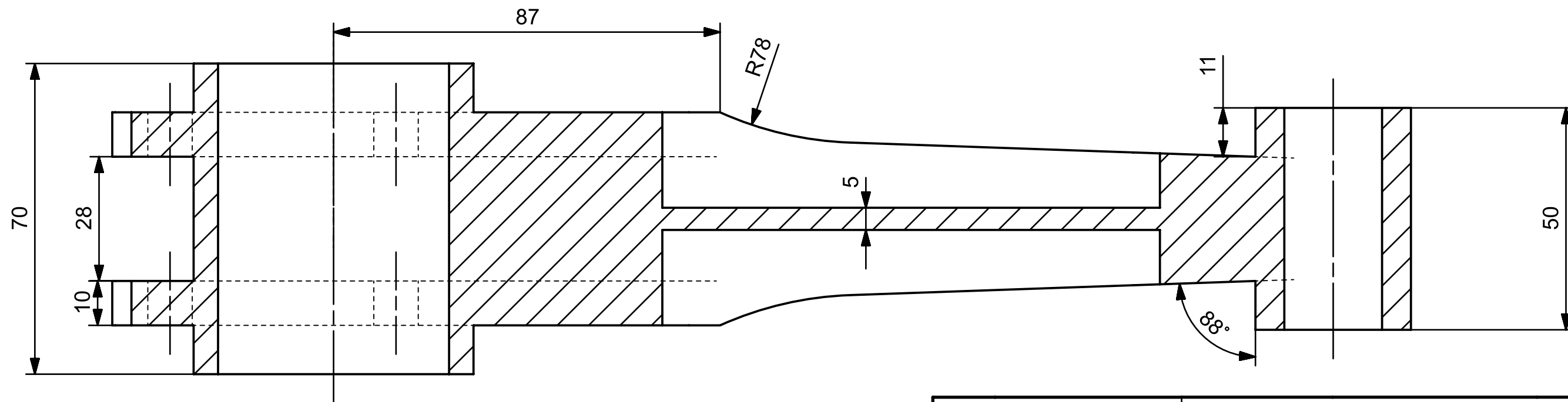
COUPE A-A
